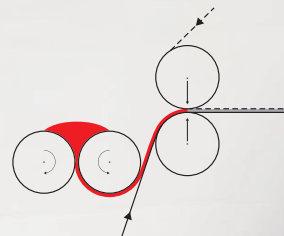
Multiroller - Gravure
